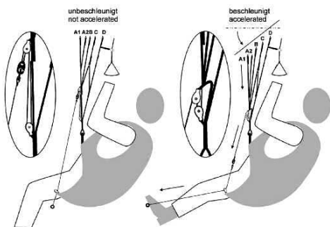
Schematische Darstellung des Beschleunigungssystems und der dadurch bedingten Veränderung der Tragegurtlängen (Swing Flugsportgeräte GmbH)
