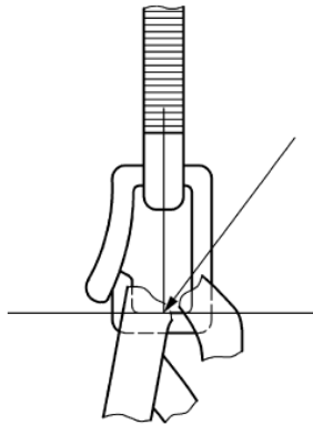
Bild 3 — Oberer Messpunkt am Gurtzeug
