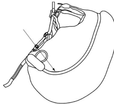
Bild 4 — Unterer Messpunkt am Gurtzeug
