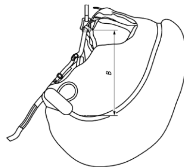
Bild 6 — Höhe der Befestigungspunkte des Gurtzeuges
