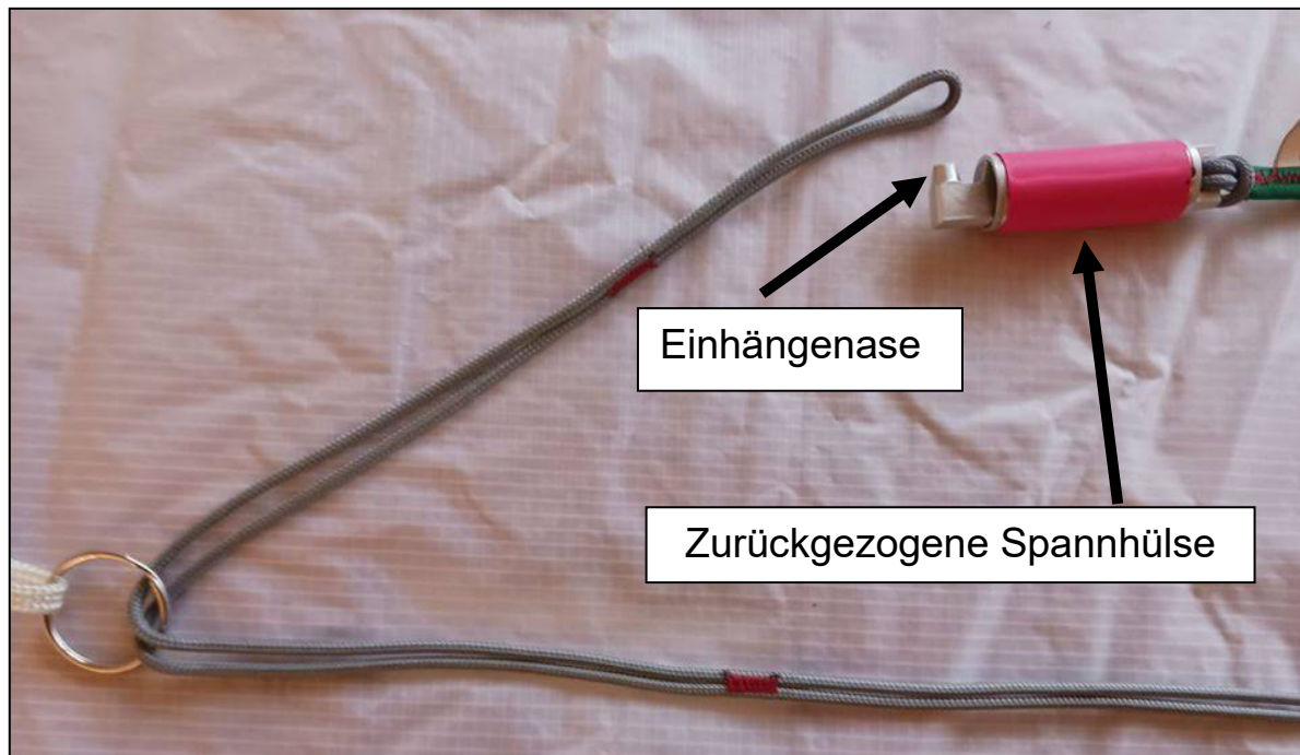
Abbildung 5.1: Spannöhse zurückgezogen
