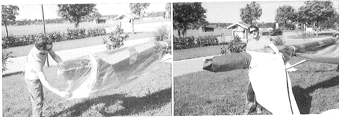
19.) Segel innen auf der Unterseite einschlagen und mittels Klettpolster am Holm fixieren
