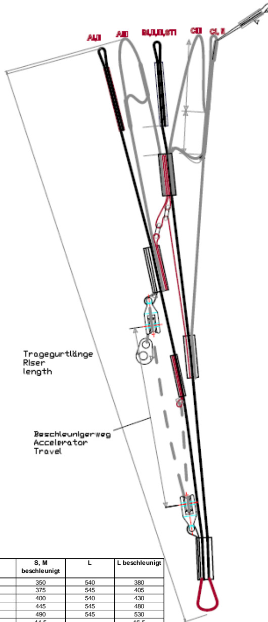
Abbildung 4: Tragegurte des UP Lhotse
