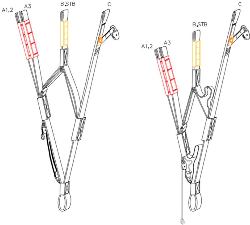
Abbildung 5: Bolero 5 Tragegurte (Trimstellung und voll beschleunigt)
