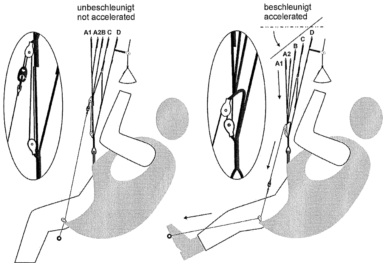
Abbildung 5: Funktionsweise Fußbeschleuniger Arcus 7
