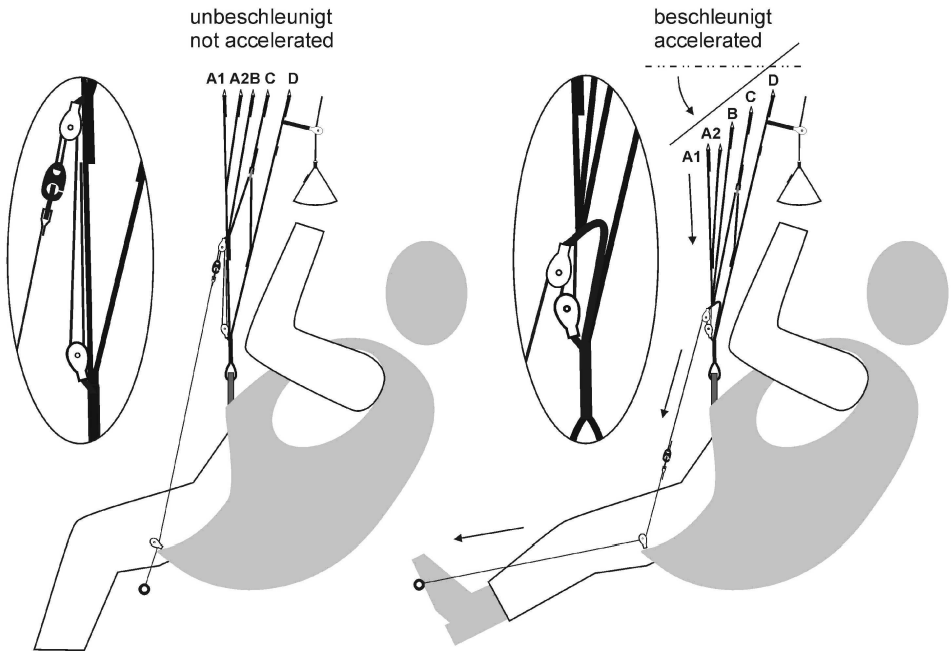
Abbildung 5: Funktionsweise Fußbeschleuniger Axis 5
