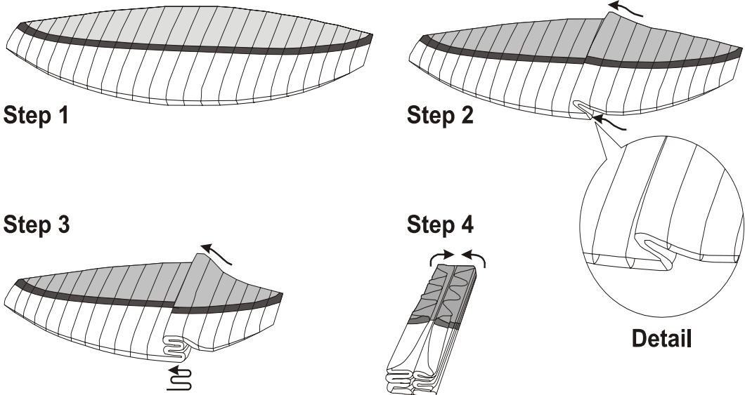
Abbildung 8: Packschritte für den UP Kantega XC
